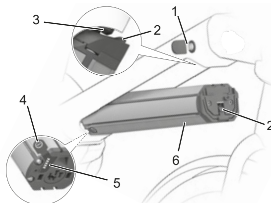
Illustration 18 : Exemple du détail d'une batterie intégrée
