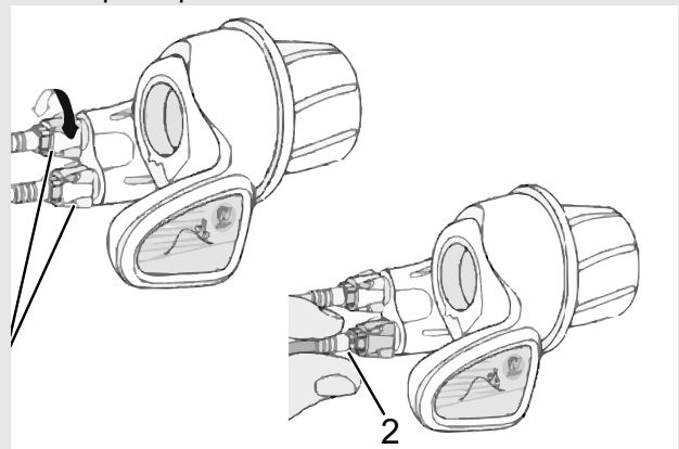
Illustration 105 : Poignée de vitesse rotative avec douilles de réglage (1) et jeu du changement de vitesse (2)
