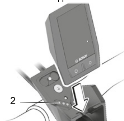
Illustration 85 : Installer l'ordinateur de bord (1)
