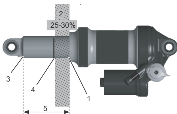
Illustration 77 : Structure d'un amortisseur arrière FOX
