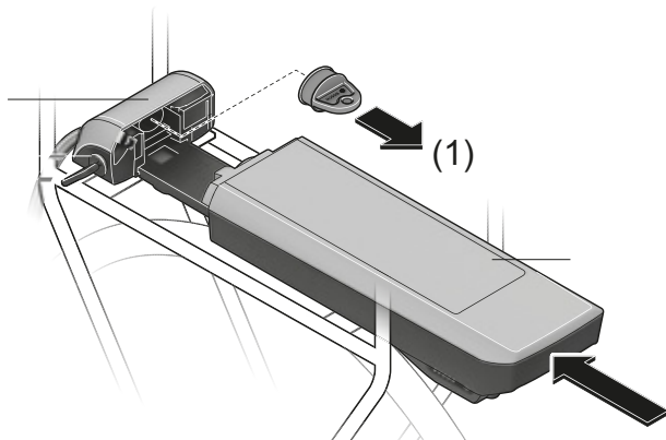
Illustration 84 : Couvrir les contacts ouverts avec un cache, exemple d'une batterie pour porte-bagages
