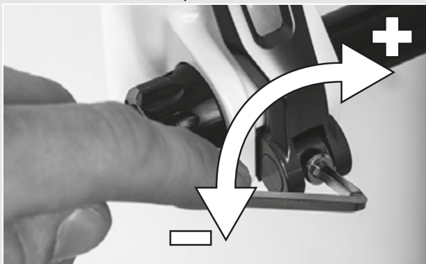
Illustration 51 : Régler la force de serrage de l'attache rapide
