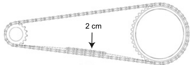
Illustration 100 : Contrôler la tension de la chaîne
