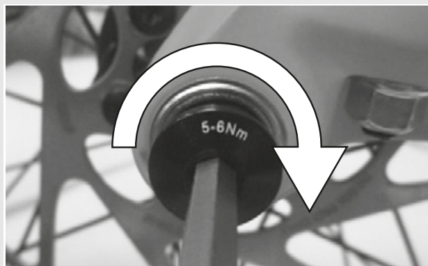
Illustration 43 : Serrer la vis de blocage
