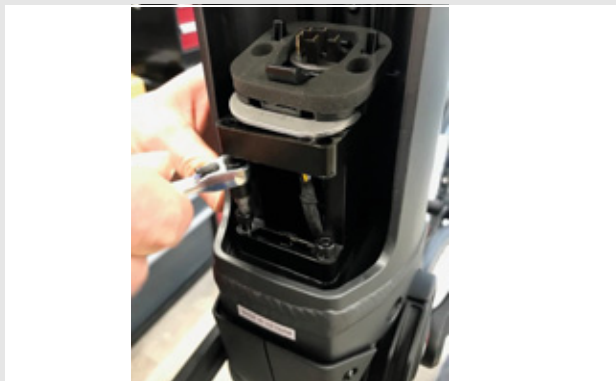
Illustration 28 : Retirer les vis à 6 pans de 4 mm
