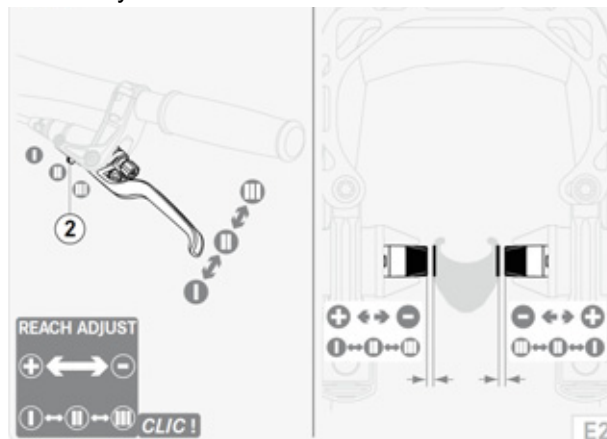
Illustration 68 : Régler la garde d'un levier de frein Magura HS22
