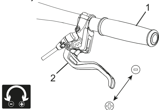
Illustration 67 : Régler la garde d'un levier de frein Magura HS33
