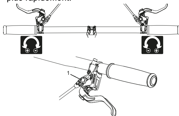
Illustration 70 : Utilisation du bouton rotatif (1) pour le réglage du point de pression
