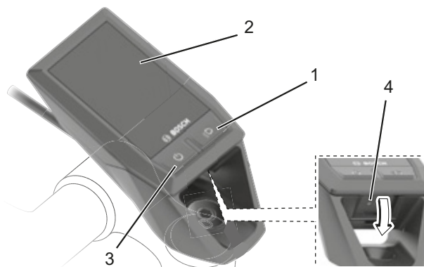
Illustration 22 : Aperçu de la structure et des éléments de commande de l'ordinateur de bord
