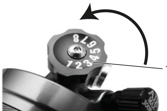
Illustration 76 : Dispositif de réglage de la compression Suntour sur l'amortisseur arrière
