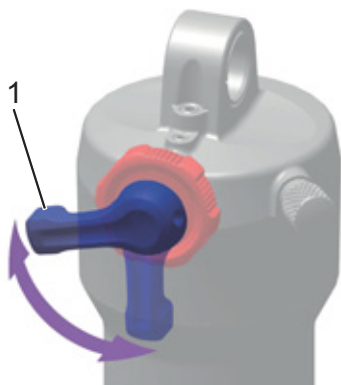
Illustration 97 : Régler la dureté de l'amortisseur de compression sur le levier de l'amortisseur (1) de l'amortisseur arrière
