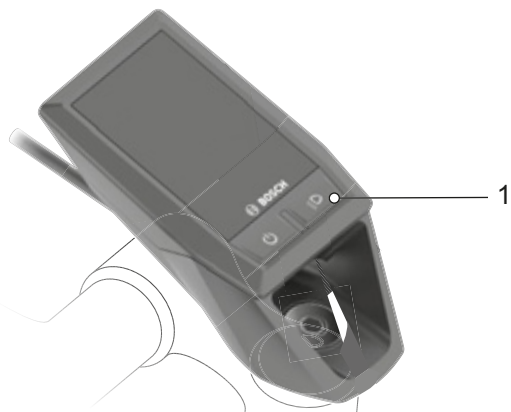
Illustration 90 : Position de la touche des feux
